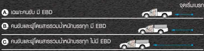
(Electronic Brake-Force Distribution) เพิ่มประสิทธิภาพการหยุดรถ ช่วยลดระยะเบรกให้สั้นลง ทำงานควบคู่กับระบบ ABS (เฉพาะรุ่น 4WD)
